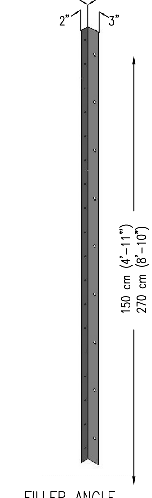
FILLER ANGLE
